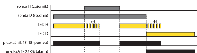
STUDNIA - ZBIORNIK, OFF DELAY (funkcje 7)
