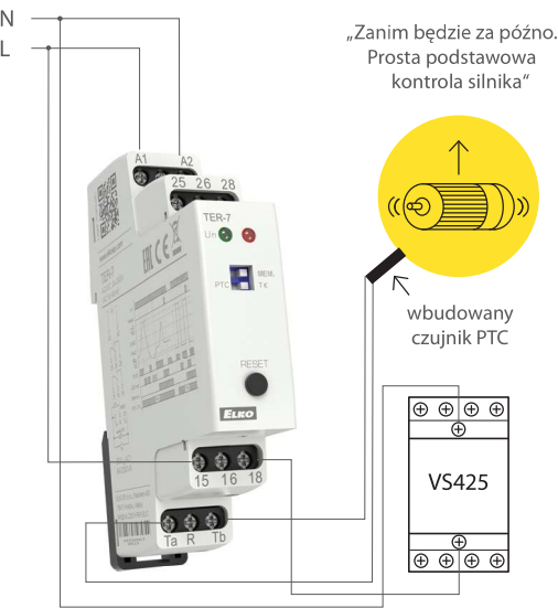
Termostat kontroli temperatury uzwojenia silnika TER-7 - ochrona silników przed przeciążeniem termicznym
