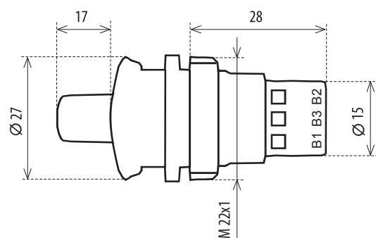
potencjometr zewnętrzny do CRM-2HE, CRM-91HE
