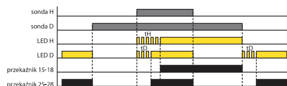
PUMP DOWN, ON DELAY (funkcje 6)
