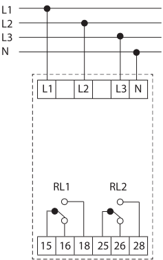
podłączenie 4-przewodowe
