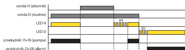
STUDNIA - ZBIORNIK, ON DELAY (funkcje 7)
