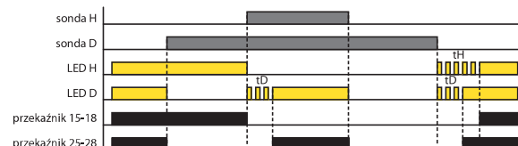
PUMP DOWN, ON DELAY (funkcje 6)
