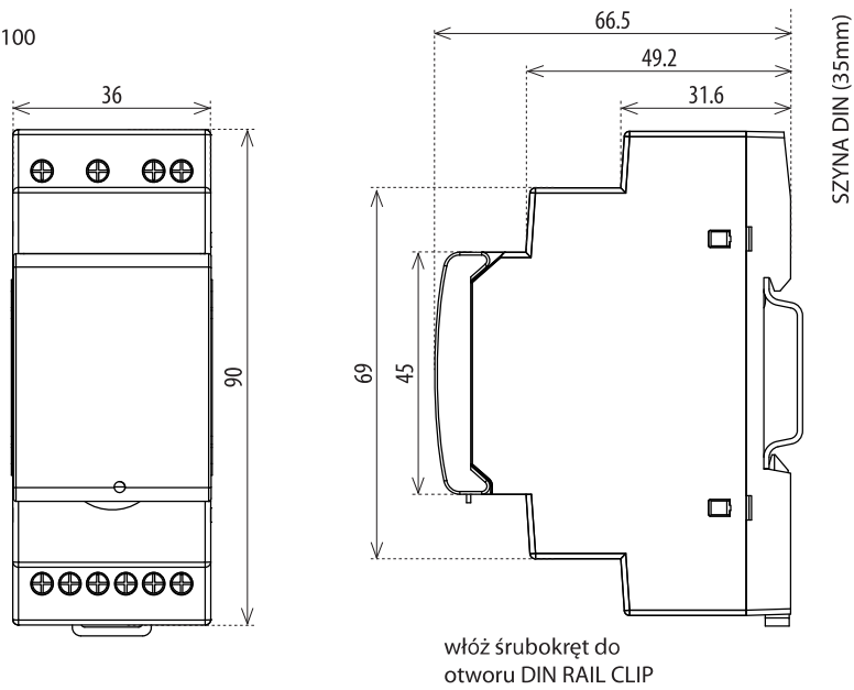
SMR-T, SMR-H, SMT-K
