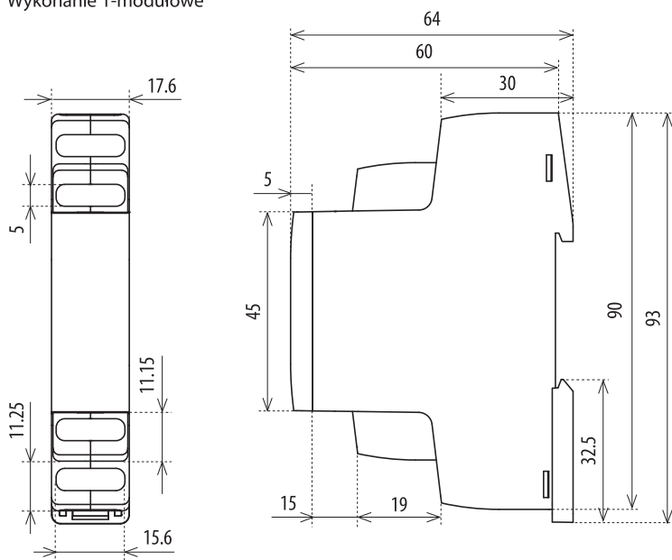
Wykonanie 1-modułowe
