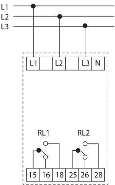
podłączenie 3-przewodowe
