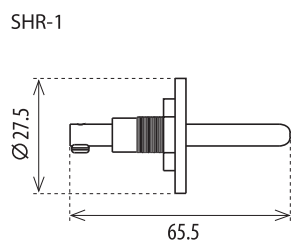
Sonda poziomu cieczy
