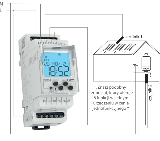
Wielofunkcyjny termostat cyfrowy TER-9 - kompleksowe sterowanie ogrzewaniem domu oraz wody
