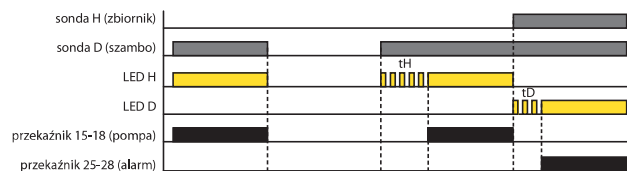
SZAMBO - ZBIORNIK, ON DELAY (funkcje 8)
