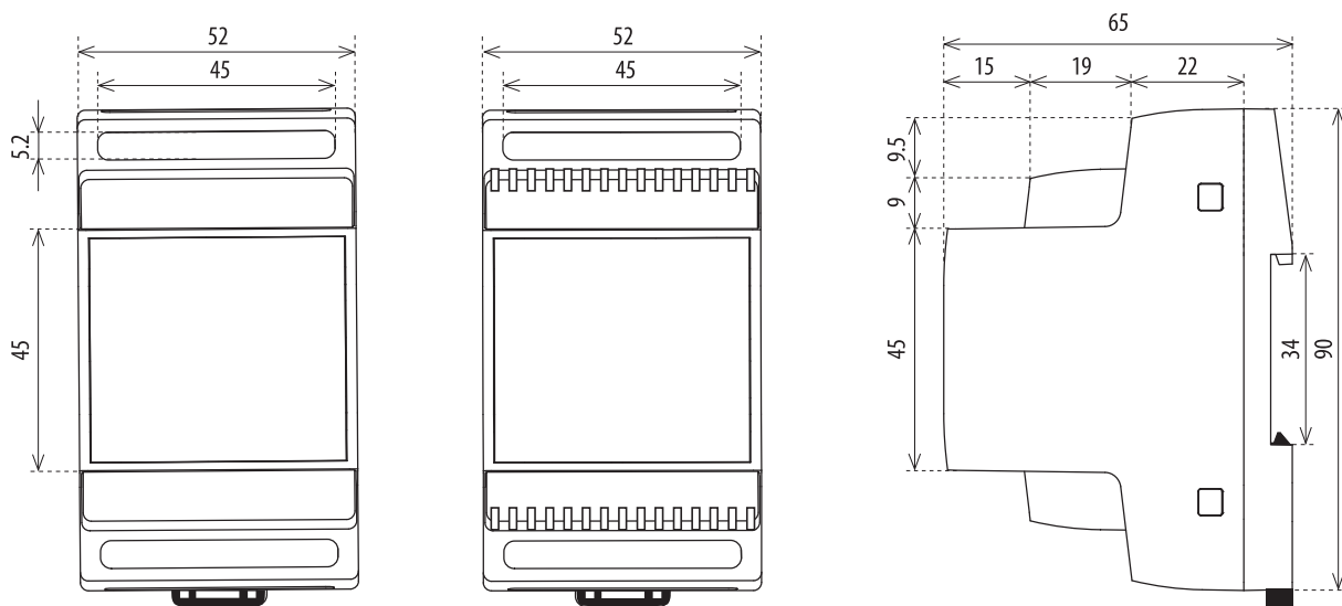
Wykonanie 3-modułowe
