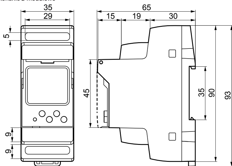
Wykonanie 2-modułowe
