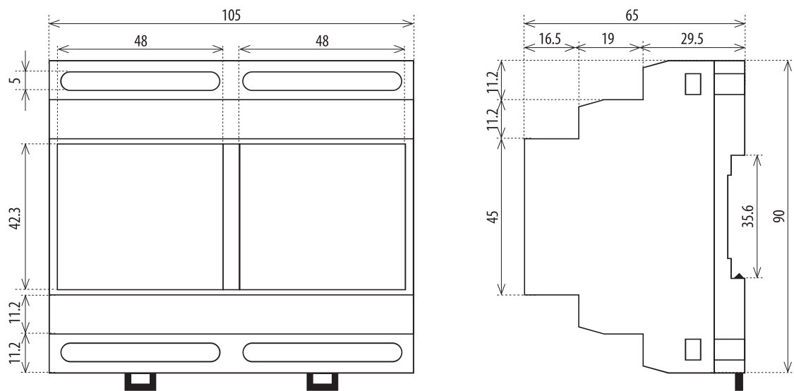
Wykonanie 6-modułowe
