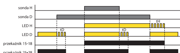
PUMP DOWN, OFF DELAY (funkcje 6)
