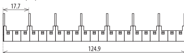
Listwa łącząca CB-17-8
